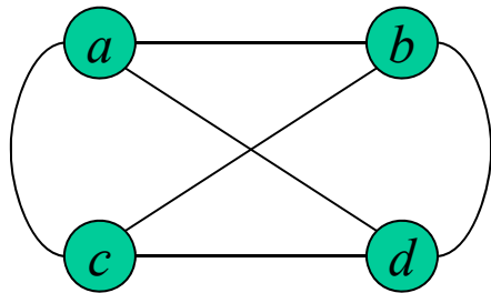
2-Opt
